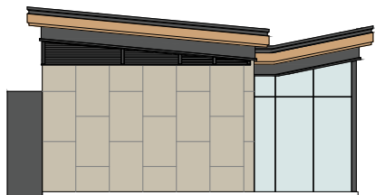
Elevation Plan D 立面圖 D
