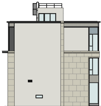
Elevation Plan C 立面圖 C (For Villa 20, 21 & 25 Only) (僅限20、21及25號洋房)
