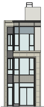
Elevation Plan E 立面圖 E
