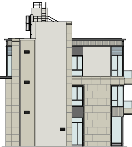
Elevation Plan H 立面圖 H
