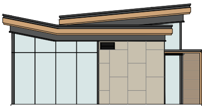
Elevation Plan C 立面圖 C
