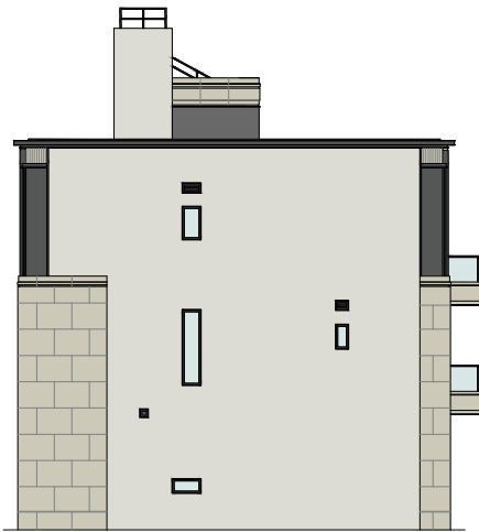
Elevation Plan C 立面圖 C
