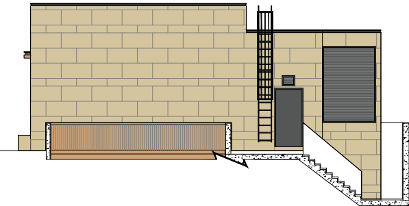
Elevation Plan E 立面圖 E
