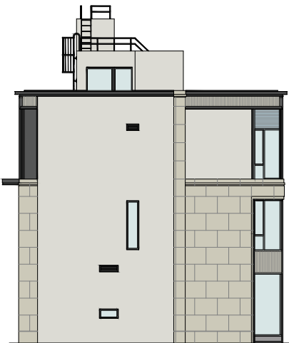
Elevation Plan C 立面圖 C (For Villa 26 Only) (只適用於26號洋房)
