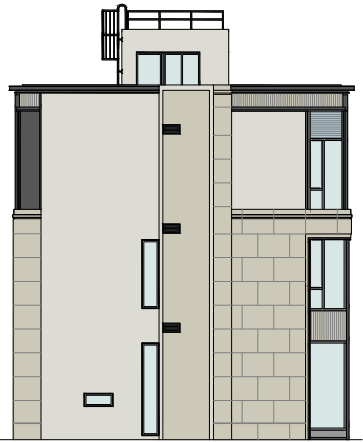
Elevation Plan F 立面圖 F
