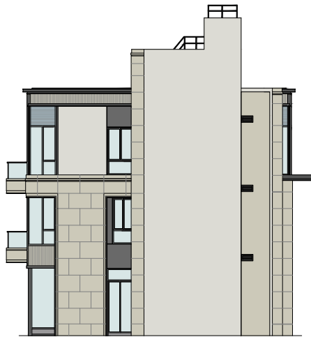
Elevation Plan C 立面圖 C
