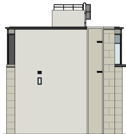
Elevation Plan D 立面圖 D (For Villa 20, 21 & 25 Only) (僅限20、21及25號洋房)
