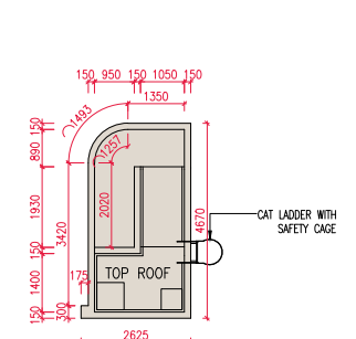
TOP ROOF PLAN 頂層天台平面圖
