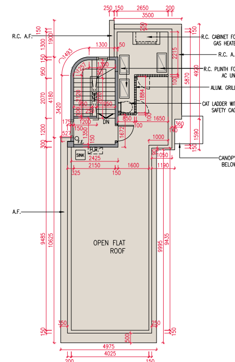
ROOF PLAN 天台平面圖
