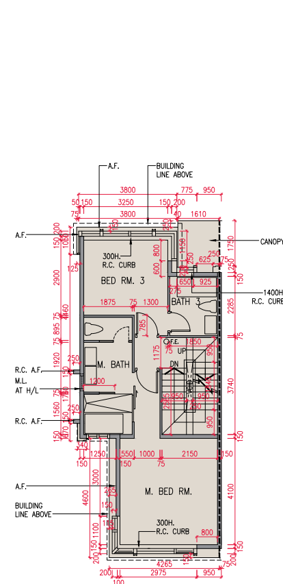
2/F PLAN 2樓平面圖
