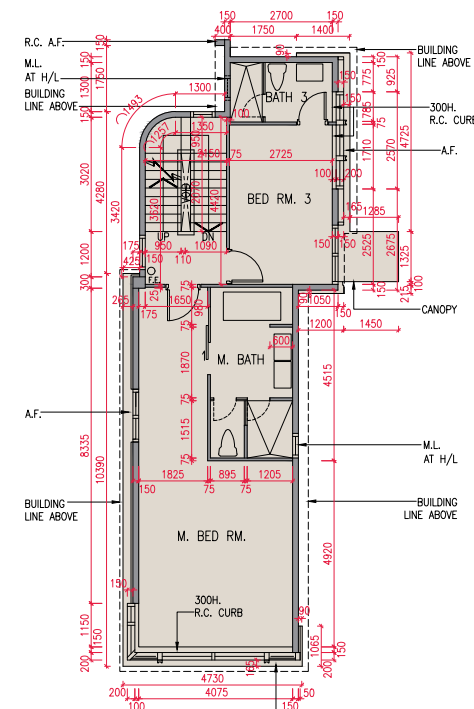
2/F PLAN 2樓平面圖
