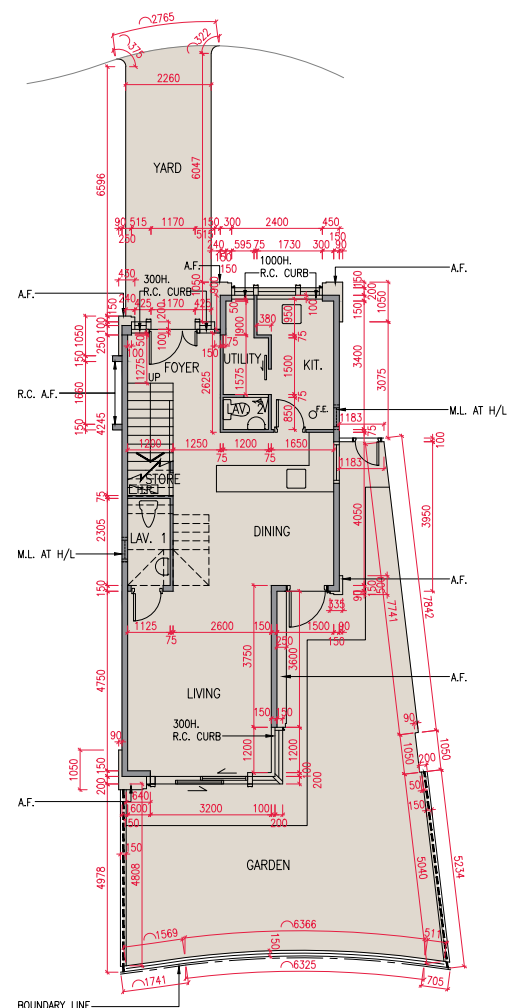
GROUND FLOOR PLAN 地下平面圖
