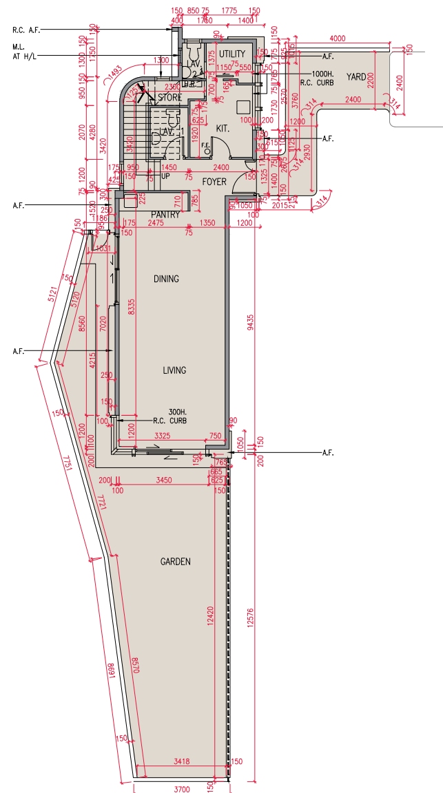
GROUND FLOOR PLAN 地下平面圖
