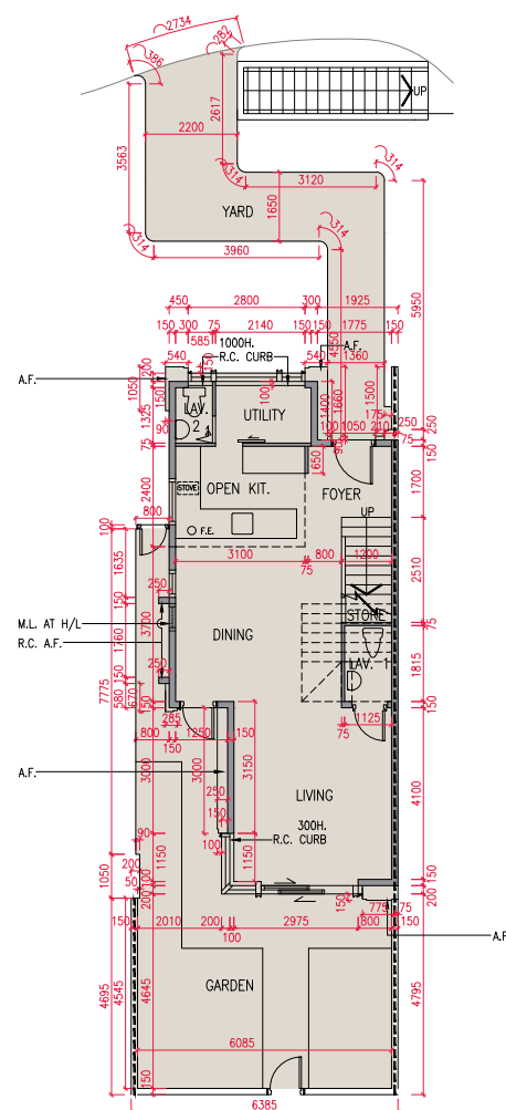
GROUND FLOOR PLAN 地下平面圖
