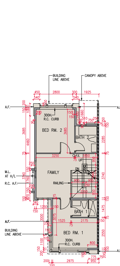
1/F PLAN 1樓平面圖
