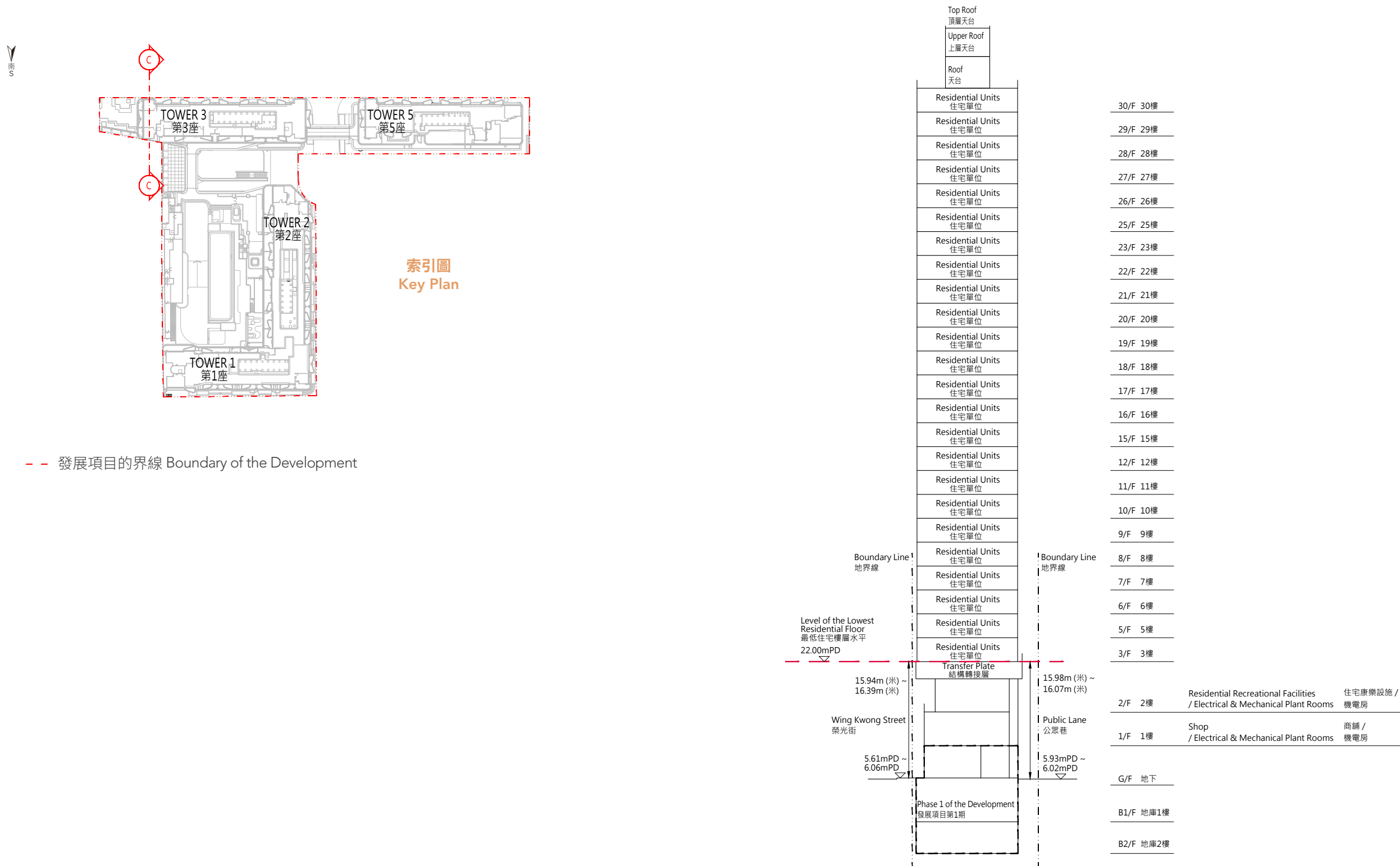
橫截面圖 C-C Cross-Section Plan C-C
