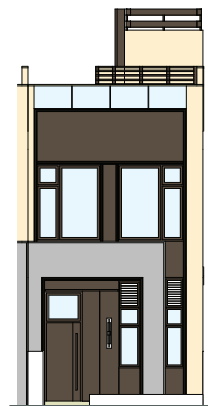
ELEVATION A 立面 A
