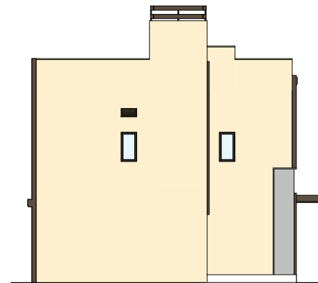
ELEVATION B 立面 B
