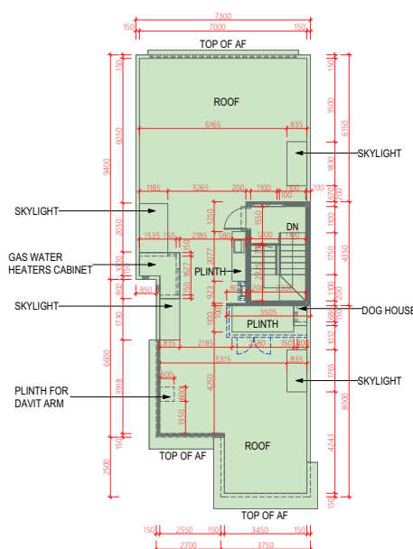
ROOF 天台
