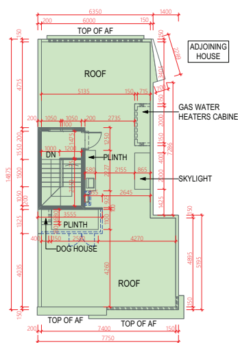
ROOF 天台
