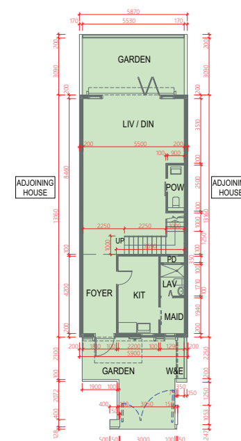
GROUND FLOOR 地下
