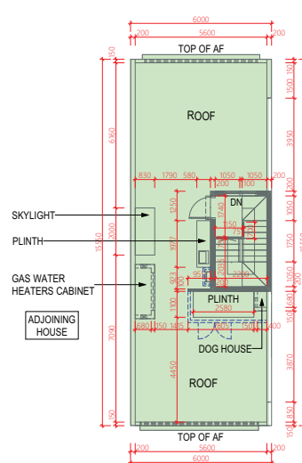
ROOF 天台
