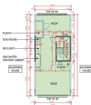
ROOF 天台
