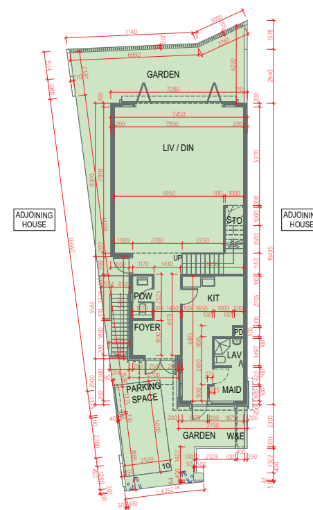
GROUND FLOOR 地下
