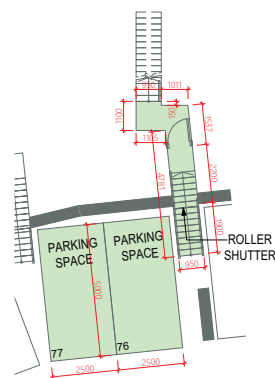
PART PLAN OF CARPARK FLOOR 停車場層部份平面圖
