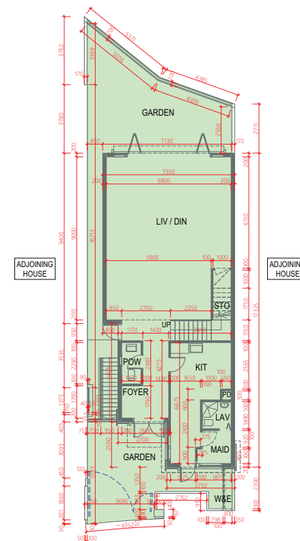
GROUND FLOOR 地下
