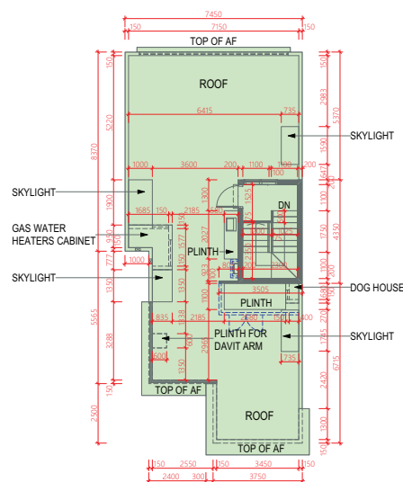
ROOF 天台
