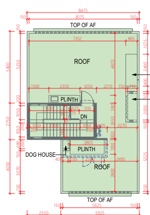
ROOF 天台
