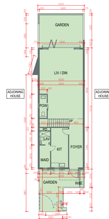
GROUND FLOOR 地下
