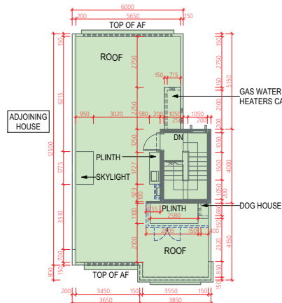
ROOF 天台
