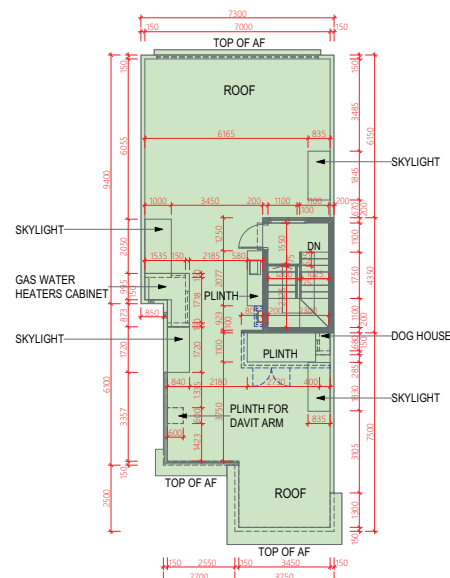
ROOF 天台
