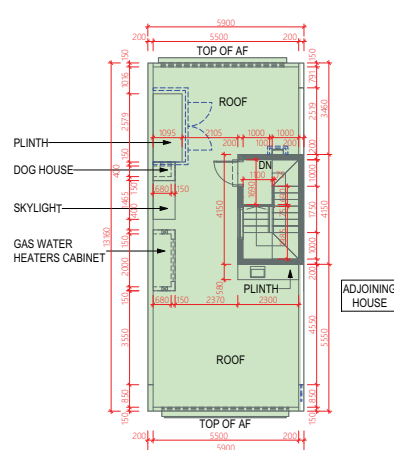
ROOF 天台
