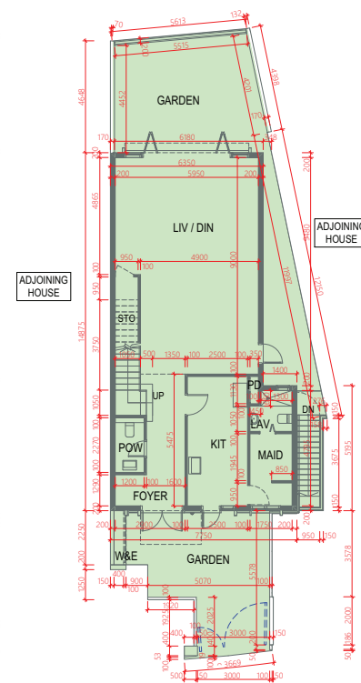
GROUND FLOOR 地下
