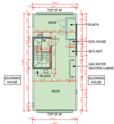
ROOF 天台
