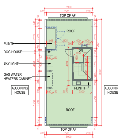
ROOF 天台
