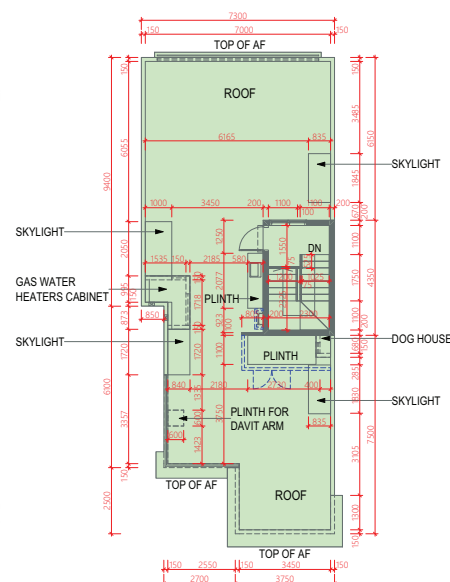
ROOF 天台
