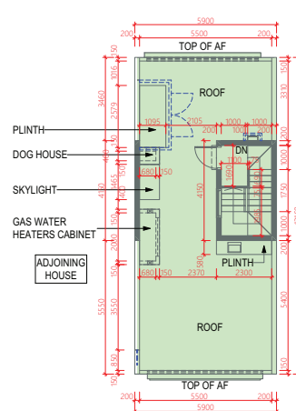
ROOF 天台
