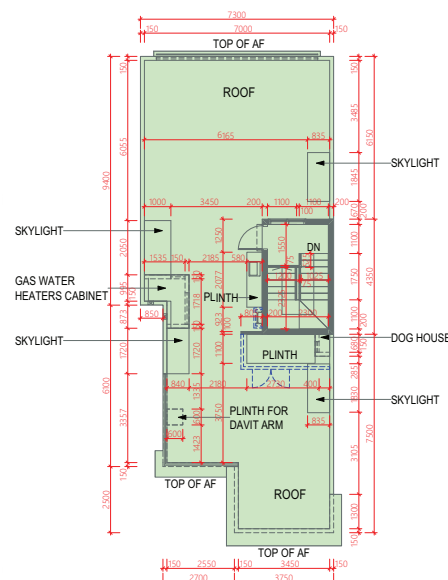
ROOF 天台
