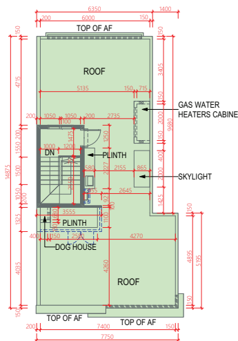
ROOF 天台
