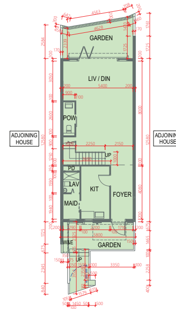
GROUND FLOOR 地下
