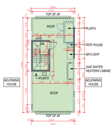
ROOF 天台
