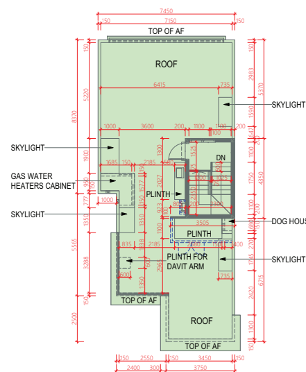
ROOF 天台
