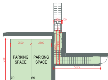
PART PLAN OF CARPARK FLOOR 停車場層部份平面圖
