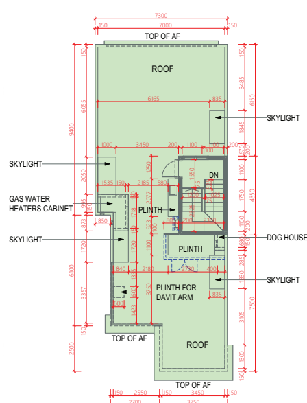
ROOF 天台
