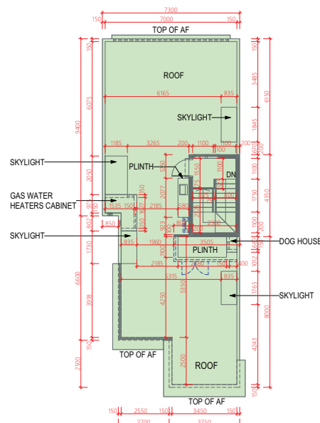
ROOF 天台
