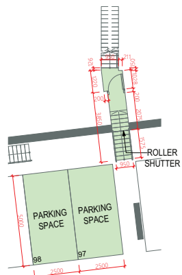
PART PLAN OF CARPARK FLOOR 停車場層部份平面圖
