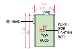
TOP ROOF 上層天台
