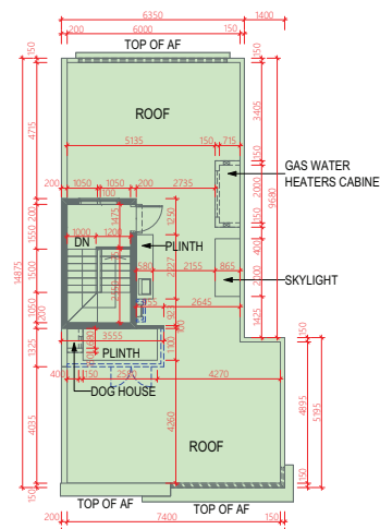
ROOF 天台
