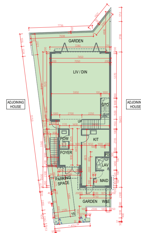
GROUND FLOOR 地下
