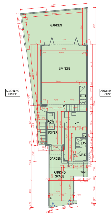
GROUND FLOOR 地下
