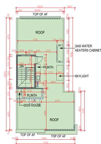
ROOF 天台
