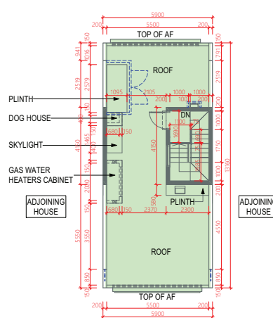
ROOF 天台
