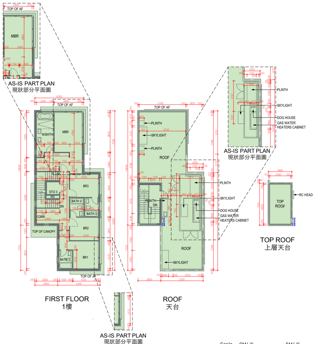
HOUSE 1 FLOOR PLAN 1號洋房樓面平面圖
