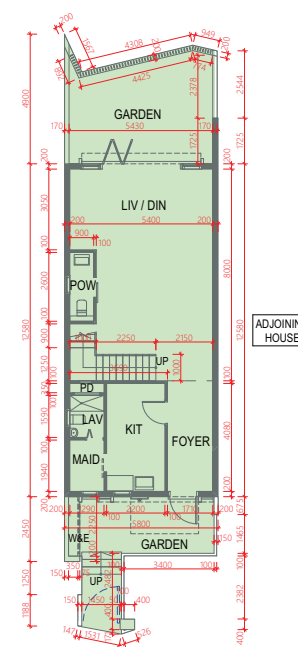
GROUND FLOOR 地下
