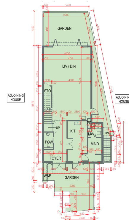
GROUND FLOOR (AS-IS PLAN) 地下 (現狀平面圖)
