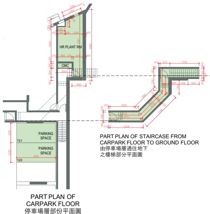
HOUSE 1 FLOOR PLAN 1號洋房樓面平面圖
