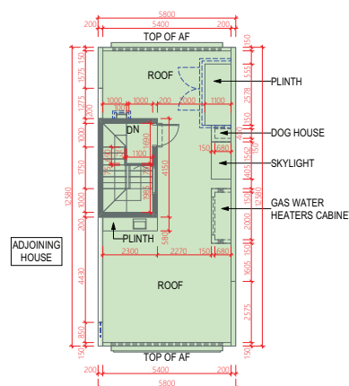
ROOF 天台
