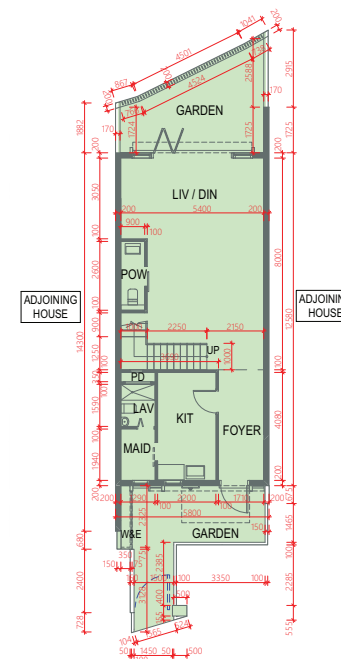
GROUND FLOOR 地下
