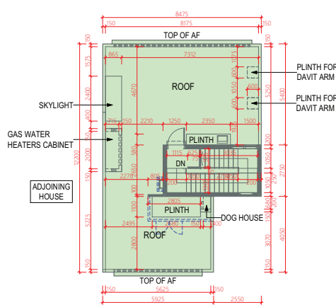
ROOF 天台
