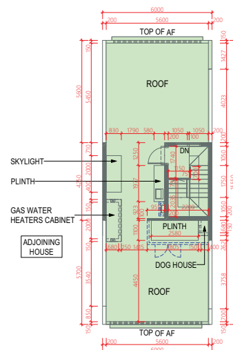
ROOF 天台
