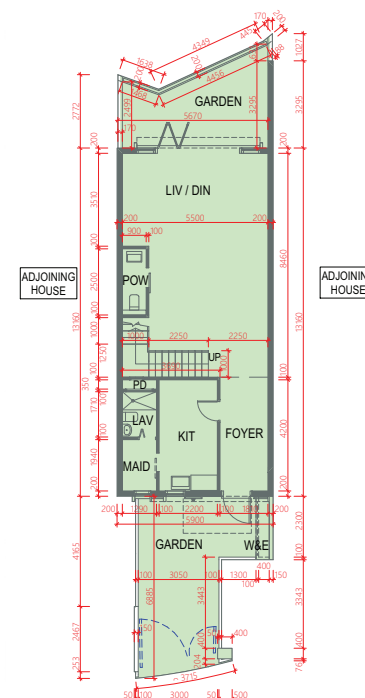
GROUND FLOOR 地下
