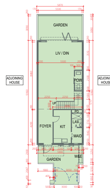
GROUND FLOOR 地下
