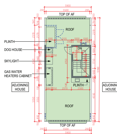
ROOF 天台
