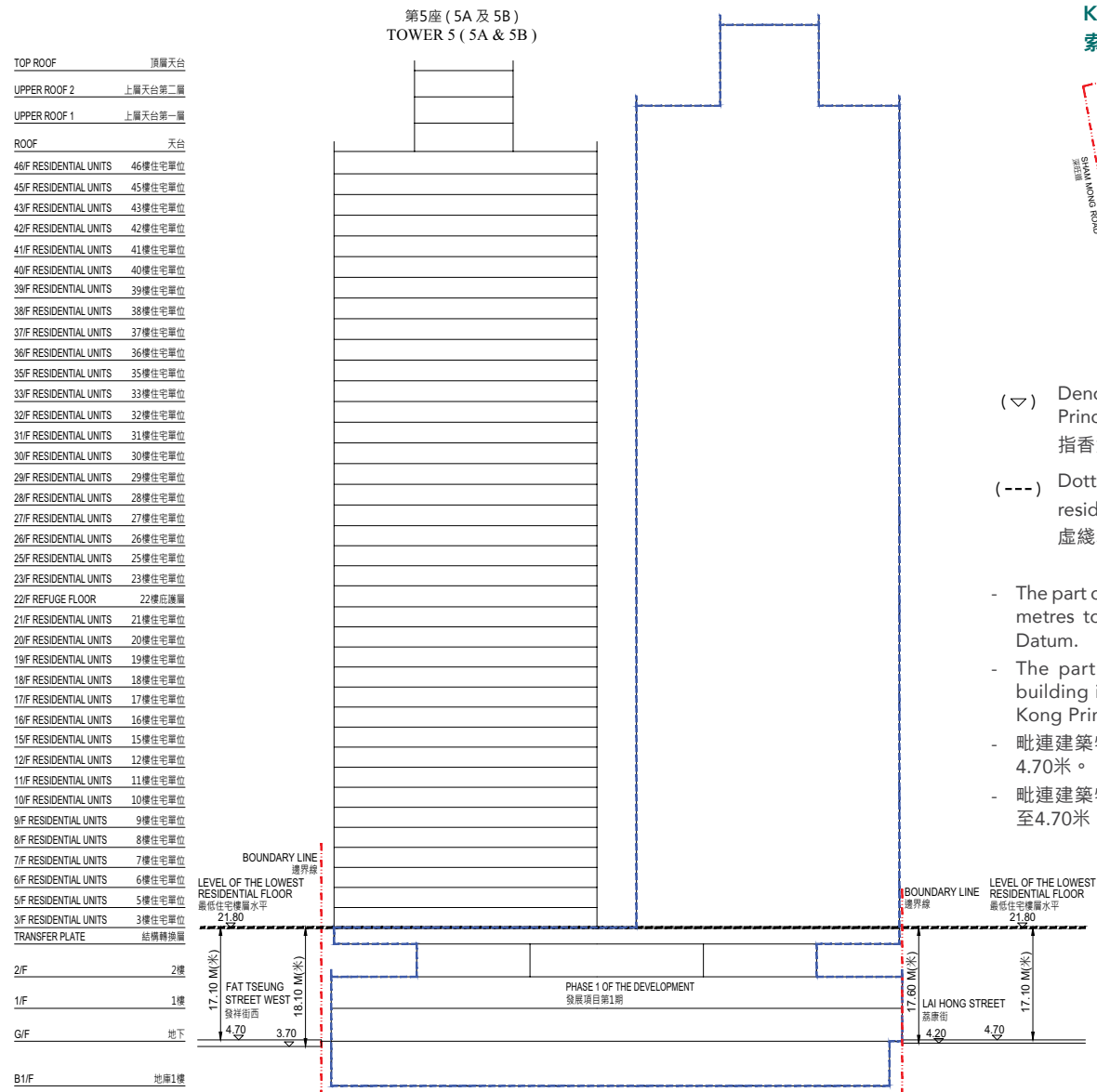
CROSS-SECTION PLAN B - B 橫截面圖 B - B
